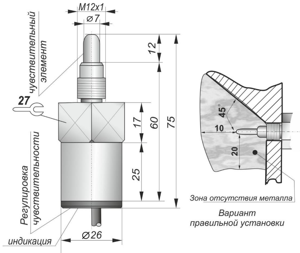
Габаритный чертеж
