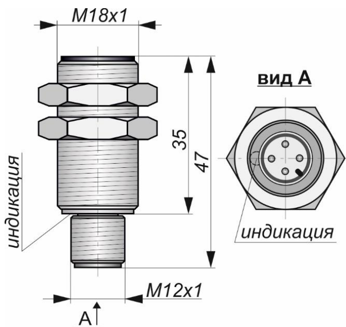
Габаритный чертеж
