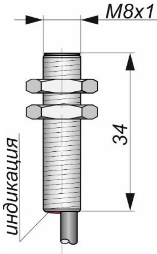
Габаритный чертеж
