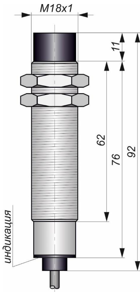
Габаритный чертеж
