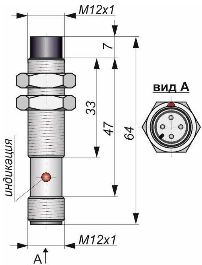
Габаритный чертеж
