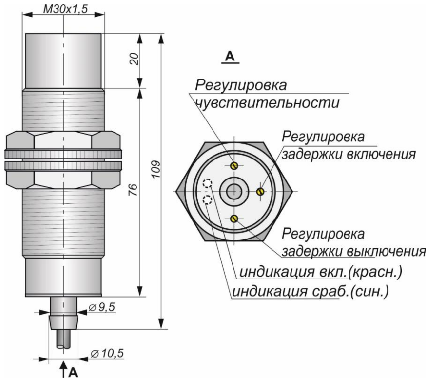
Габаритный чертеж
